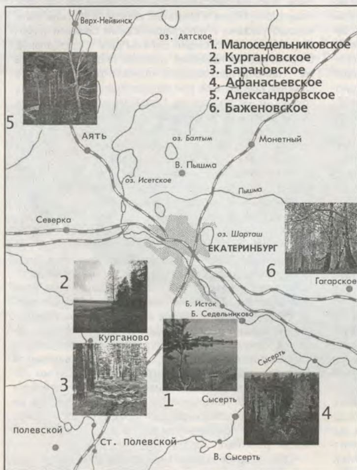
Месторождения и рудопроявления родонита на Среднем Урале:
